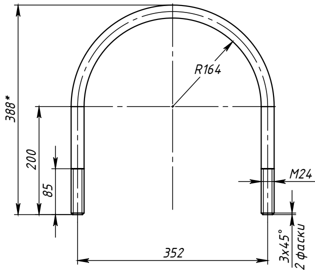
Поз.5 (Хомут)
