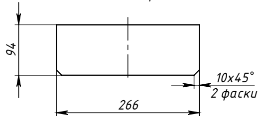
Поз.2 (Ребро)
